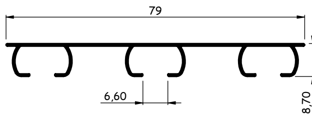
AL753 0,283 - 0,347 kg/m AL753B 0,264 - 0,322 kg/m
