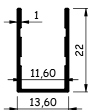
AL555 (PU-344) 0,182 - 0,223 kg/m
