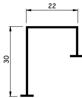
AL001M 0,107 - 0,131 kg/m
