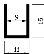
AL836 0,315 - 0,385 kg/m
