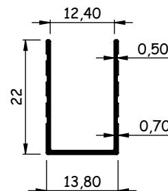
AL076 0,091 - 0,111 kg/m
