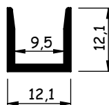
AL835 0,102 - 0,124 kg/m
