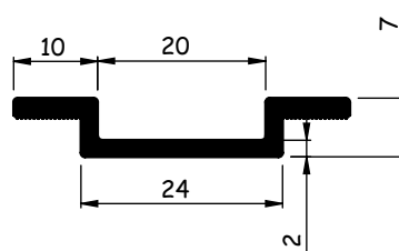
AL190 0,252 - 0,308 kg/m
