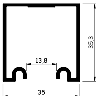
AL065 (DS-266) 0,438 - 0,535 kg/m
