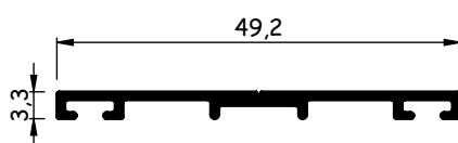
AL931 0,275 - 0,305 kg/m
