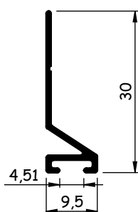
AL264 (DS-264) 0,077 - 0,095 kg/m
