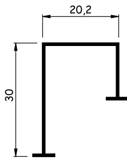
AL001L 0,108 - 0,132 kg/m
