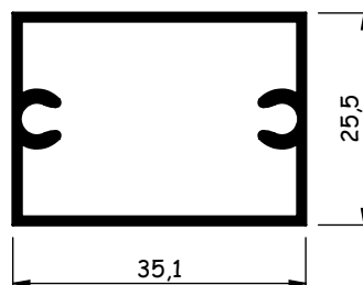
AL2535 0,461 - 0,563 kg/m
