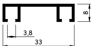
AL727 0,159 - 0,194 kg/m
