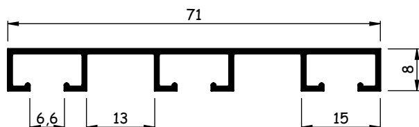
AL722 0,285 - 0,348 kg/m
