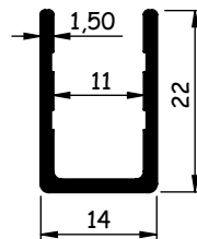
AL838P 0,193 - 0,235 kg/m
