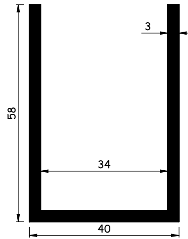
AL152 0,042 - 0,052 kg/m
