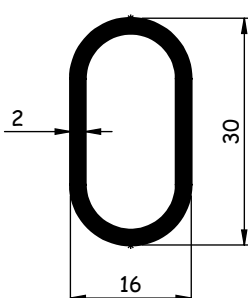
AL1001P 0,350 - 0,428 kg/m
