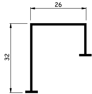
AL001P 0,147 - 0,180 kg/m
