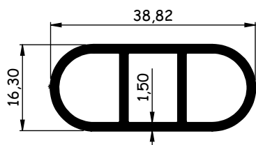
AL1005 0,169 - 0,206 kg/m
