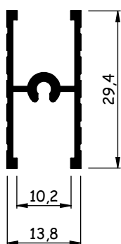
AL049C (BX-159) 0,200 - 0,245 kg/m
