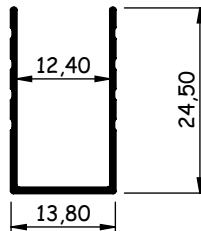
AL074 0,099-0,122 kg/m
