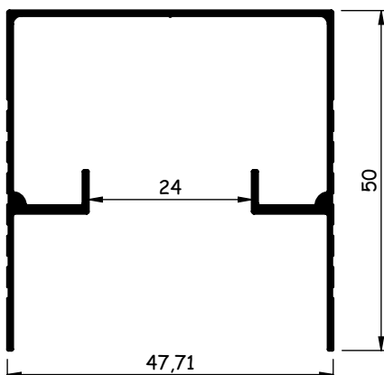
AL041C-P 0,366 - 0,448 kg/m
