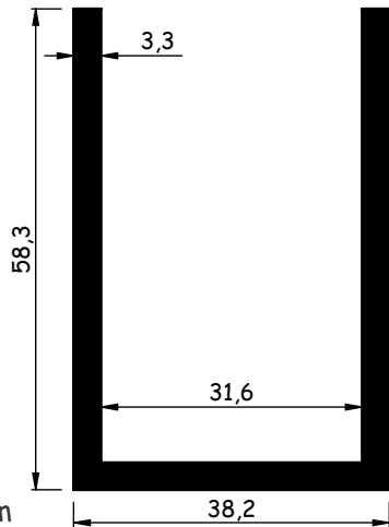
AL074 0,099-0,122 kg/m
