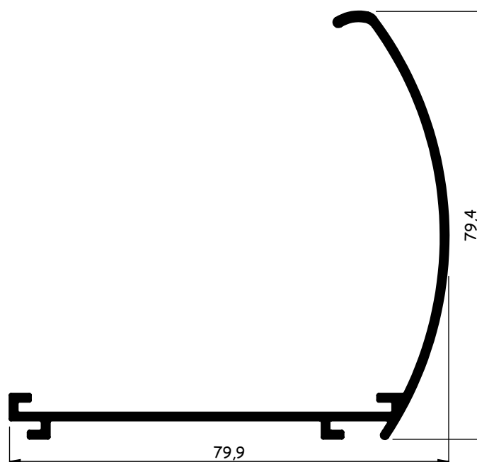
AL758 0,684 - 0,836 kg/m
