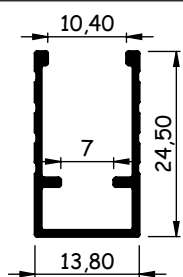
AL046C (BX-158) 0,153 - 0,176 kg/m AL046C-L 0,130 - 0,152 kg/m
