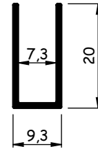
AL152 0,042 - 0,052 kg/m
