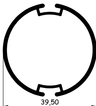
AL757L 0,346 - 0,426 kg/m AL757P 0,427 - 0,526 kg/m
