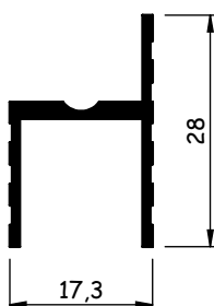
AL068C (BX-106) 0,183 - 0,223 kg/m
