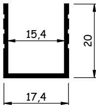
AL069 (BX-112) 0,128 - 0,156 kg/m
