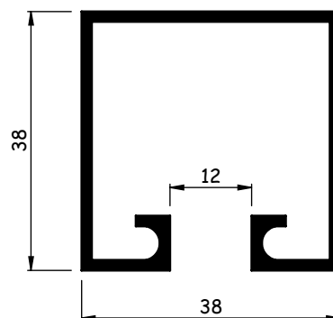
AL066 (DS-152) 0,573 - 0,701 kg/m
