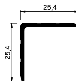
AL6017 0,232 - 0,284 kg/m
