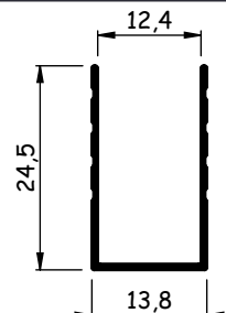
AL074 0,099 - 0,121 kg/m
