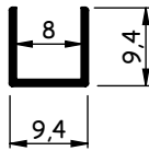
AL036 0,045 - 0,055 kg/m
