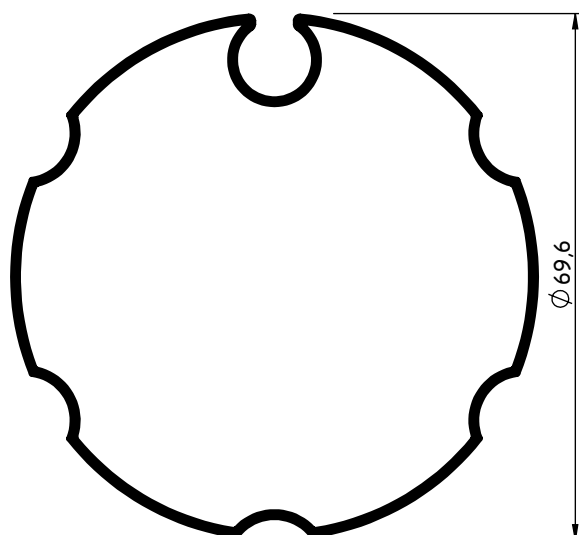
AL904 0,656 - 0,802 kg/m
