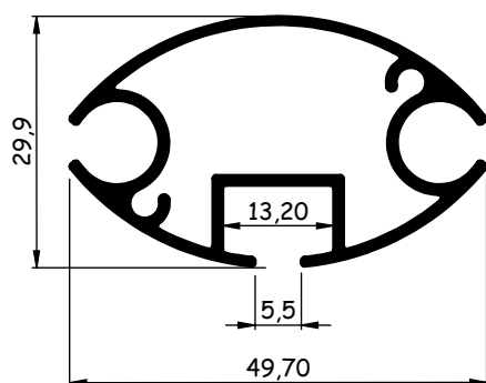
AL906 0,553 - 0,676 kg/m
