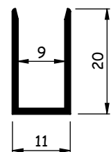
AL841 0,125-0,145 kg/m
