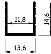
AL062 0,087 - 0,106 kg/m
