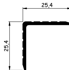
AL6003 0,176 - 0,215 kg/m
