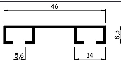
AL721 0,214 - 0,261 kg/m
