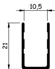
AL046C (BX-158) 0,153 - 0,176 kg/m AL046C-L 0,130 - 0,152 kg/m
