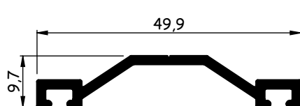
AL267 0,137 - 0,167 kg/m
