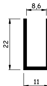
AL069 0,128 - 0,156 kg/m
