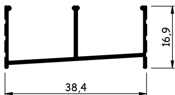
AL031C-L 0,164 - 0,200 kg/m
