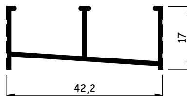
AL031C-P (BX-175) 0,220 - 0,269 kg/m
