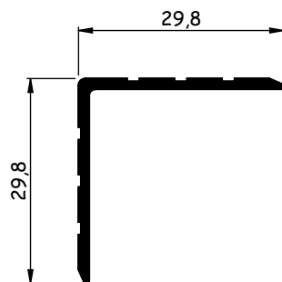
AL6006 0,195 - 0,239 kg/m
