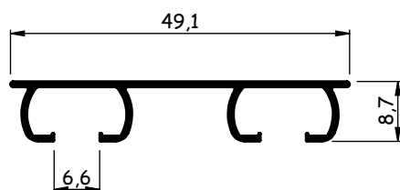
AL752 0,182 - 0,222 kg/m AL752B 0,228 - 0,279 kg/m
