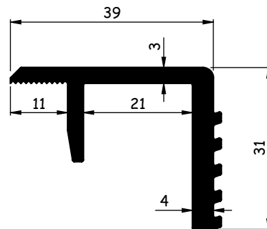
AL7013 0,683 - 0,835 kg/m
