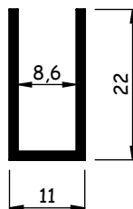
AL835 0,102 - 0,124 kg/m
