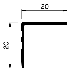
AL6020 0,078 - 0,096 kg/m
