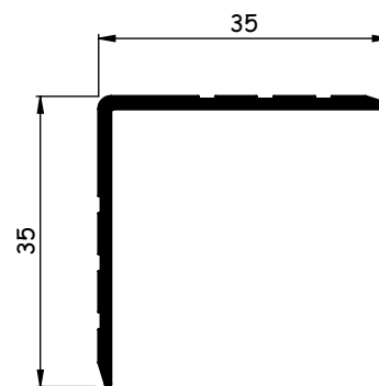
AL6017 0,232 - 0,284 kg/m
