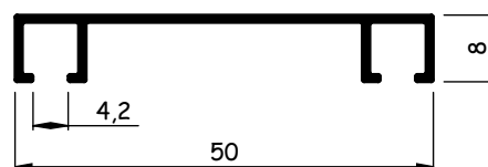
AL728 0,181 - 0,222 kg/m
