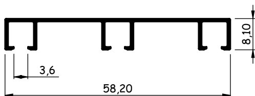
AL729 0,214 - 0,261 kg/m
