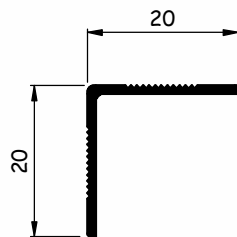
AL6011 0,110 kg/m
