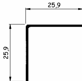
AL6004 0,148 kg/m
