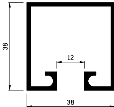
AL066 (DS-152) 0,640 kg/m
