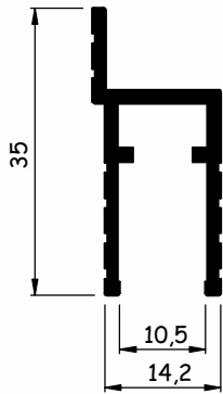
AL6007 0,319 kg/m
