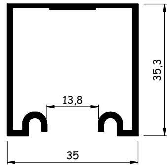
AL065 (DS-266) 0,490 kg/m
