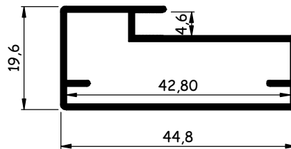
AL1517 (BK-517) 0,489 kg/m
