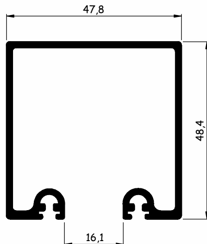
AL823 0,873 kg/m
