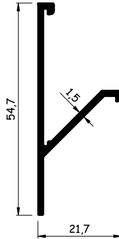
AL1534 0,353 kg/m
