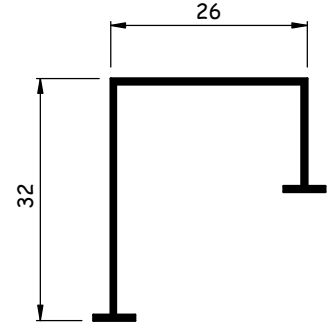
AL001P 0,160 kg/m
