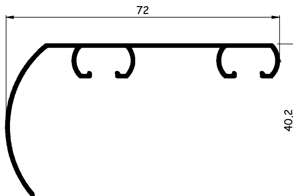
AL754 0,330 kg/m
