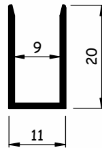
AL841 0,125-0,145 kg/m
