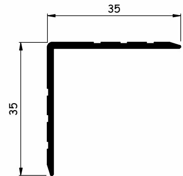
AL6017 0,258 kg/m
