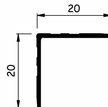
AL6020 0,087 kg/m
