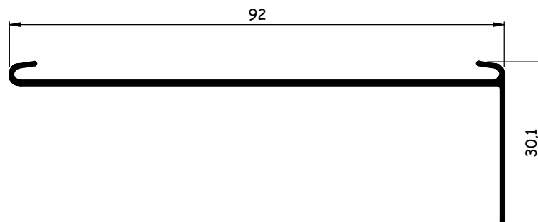
AL111L 0,265-0,300 kg/m
