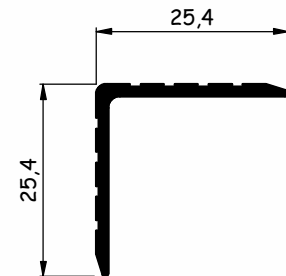
AL6003 0,200 kg/m
