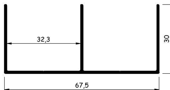
AL1519 0,420 kg/m
