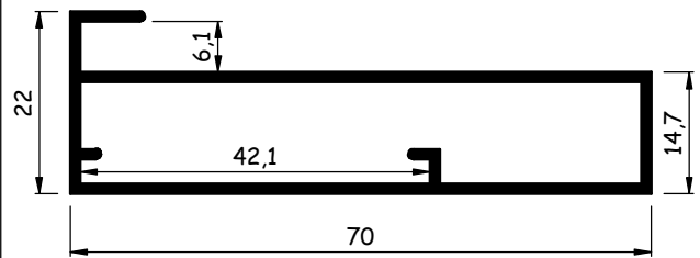
0,610 kg/m
