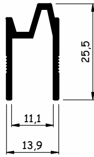
AL6005 0,238 kg/m
