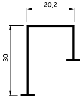
AL001L 0,115 kg/m
