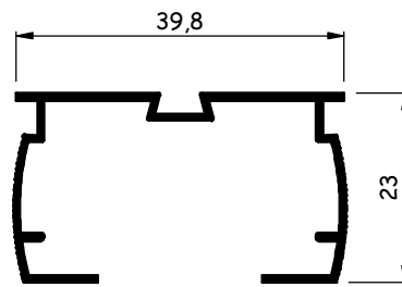
AL733 0,112 kg/m
