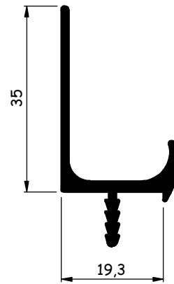
AL1505 0,320 kg/m
