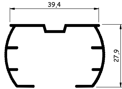
AL064 0,250-0,285 kg/m
