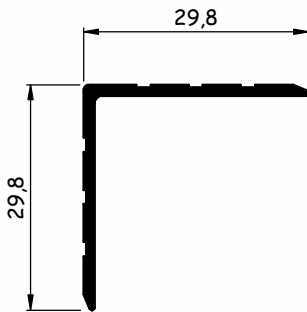
AL6006 0,217 kg/m
