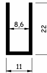
AL342 1,32 kg/m
