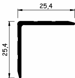
AL6021 0,189 kg/m
