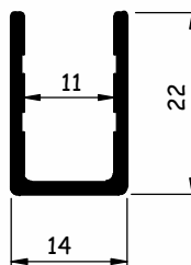
AL838L 0,125 - 0,145 kg/m AL838P 0,155 - 0,180 kg/m
