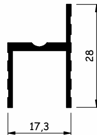
AL031C-P (BX-175) 0,250 kg/m
