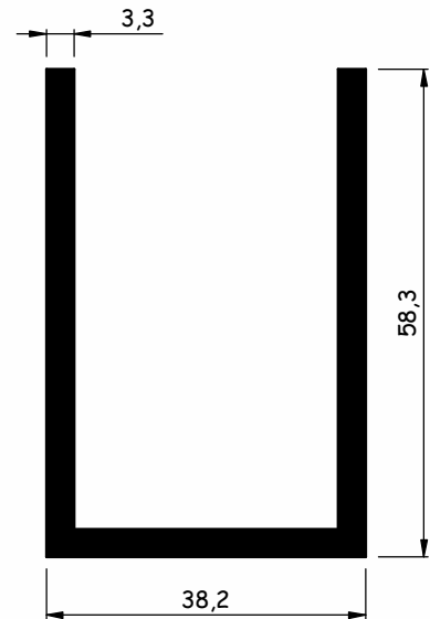
AL342 1,32 kg/m
