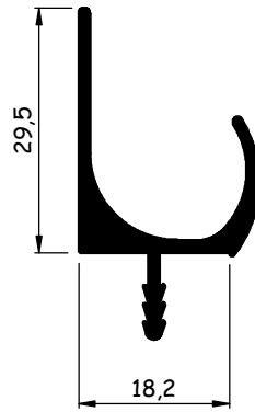
AL1527 0,376 kg/m
