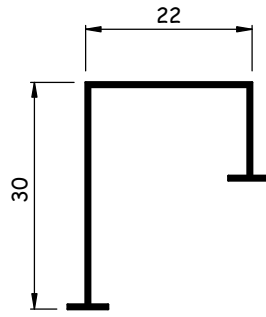
AL001M 0,119 kg/m
